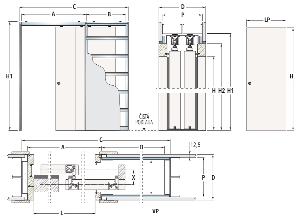
STANDARDNÍ MODEL
